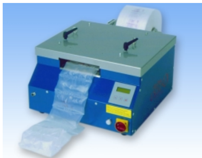
MarkII Luftkissensystem
